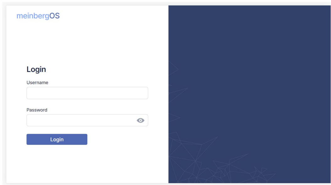
Abbildung 10.1: meinbergOS-Webinterface – Login-Seite
