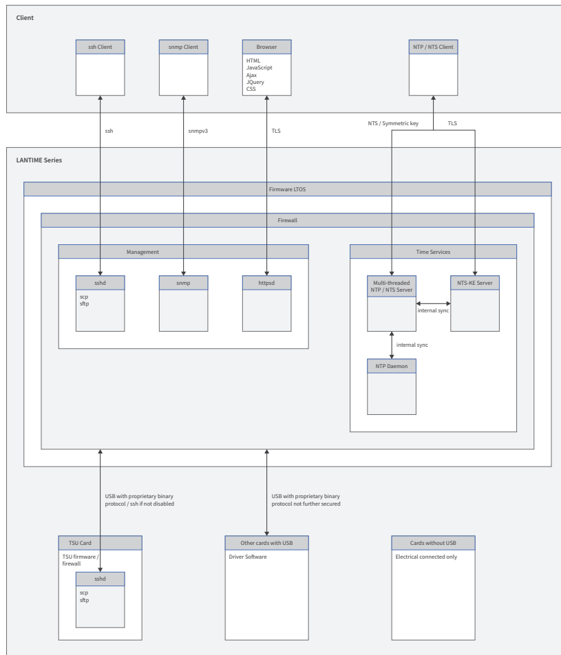
Abbildung 8.2: Die sicheren Protokolle im Detail
