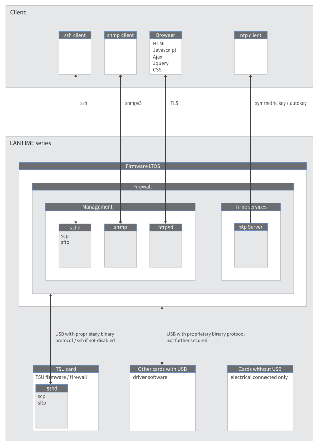
Abbildung 7.2: Die sicheren Protokolle im Detail
