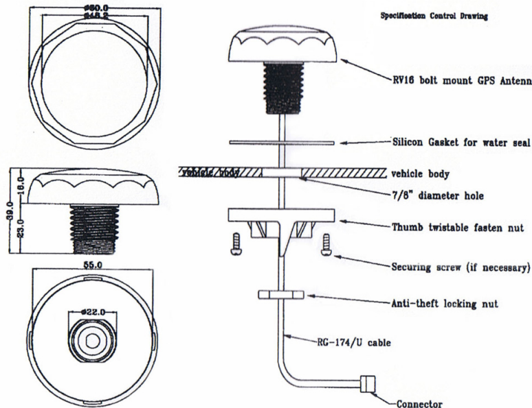
Abbildung: Montagezeichnung RV-76G Antenne
