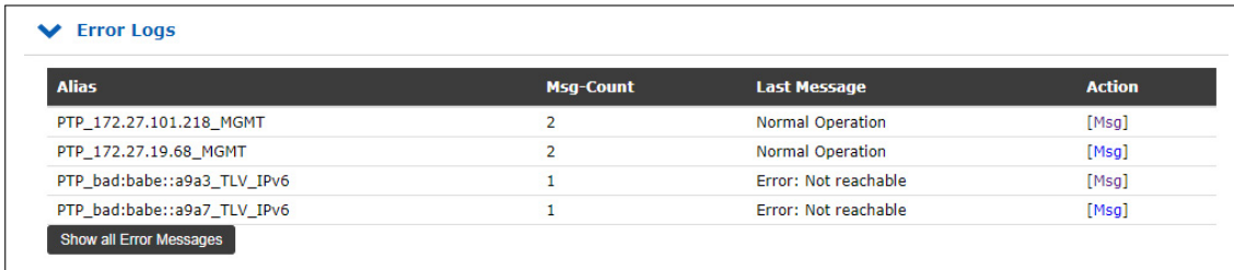
Abbildung: Fehlerprotokoll-Statistik.
