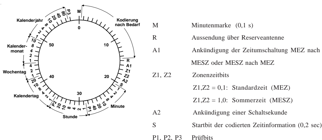
Abb.: Decodierschema
