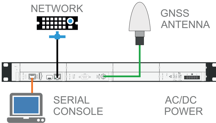
Abbildung: Anschlussschema LANTIME M1000 mit Spannungsversorgung, Netzwerkanschluss, seriellen Terminalanschluss und Antennenanschluss
